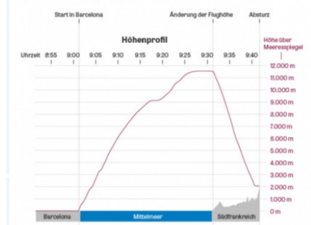
Germanwings-Flug 4U9525: Höhe und Geschwindigkeit
